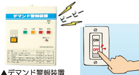
▲デマンド警報装置
