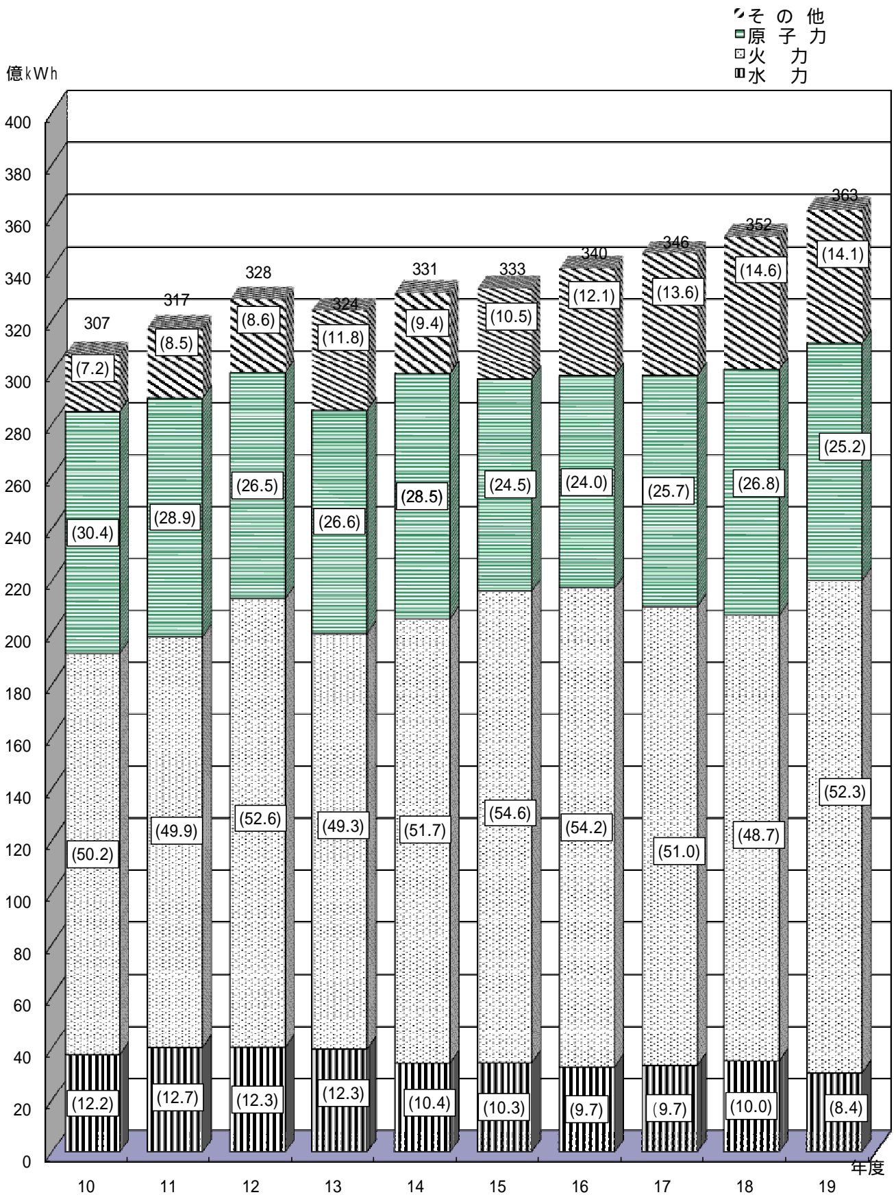
【参考 - 4】 一般電気事業者供給力（発受電力量実績）の推移
