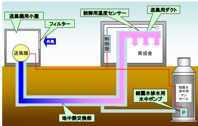
▲地中熱交換システム
