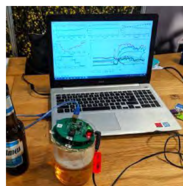
ビールの品質検査デバイス
