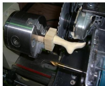
【3D加工例】
