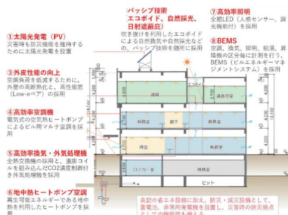
▲美幌町新庁舎 ZEB化技術
