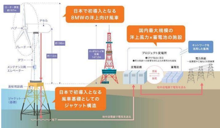
▲石狩湾新港洋上風力発電所概要図
