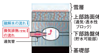
融雪模式図
