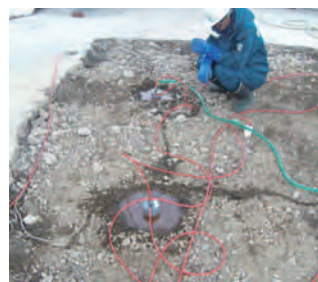
パイプ表面に開けた小さな穴からバイオ製剤が地中に染み出して広がっていく
